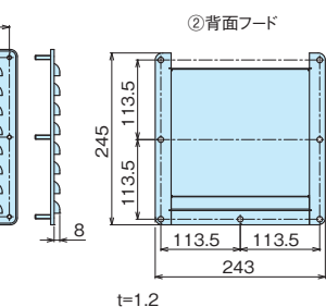
HVT-2525CA-F
