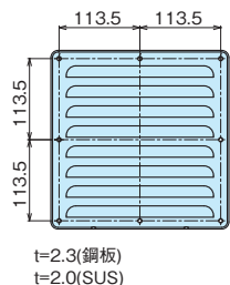
HVT-2525S-F ①通気ルーバー
