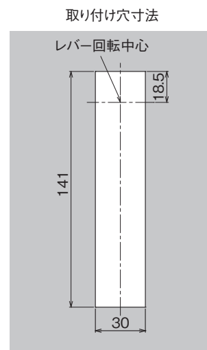
適用扉板厚は、t1.5~3.2mm
